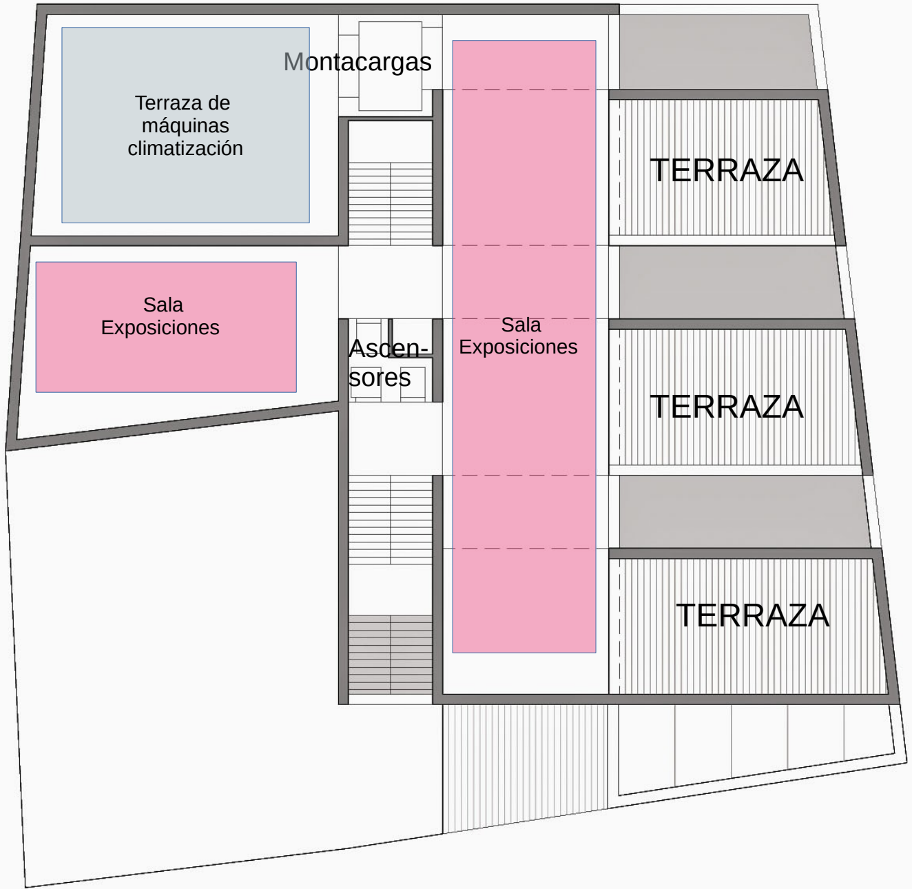
PLANTA TERCERA (+14.25)
