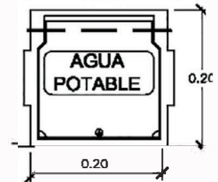
DETALLE TRAMPILLA LLAVE REGISTRO
