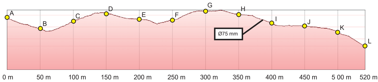
Diámetro tubería por tramo
