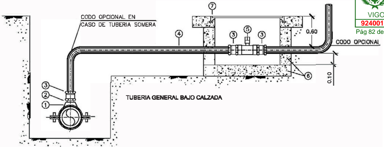
DETALLE TRAMPILLA LLAVE REGISTRO
