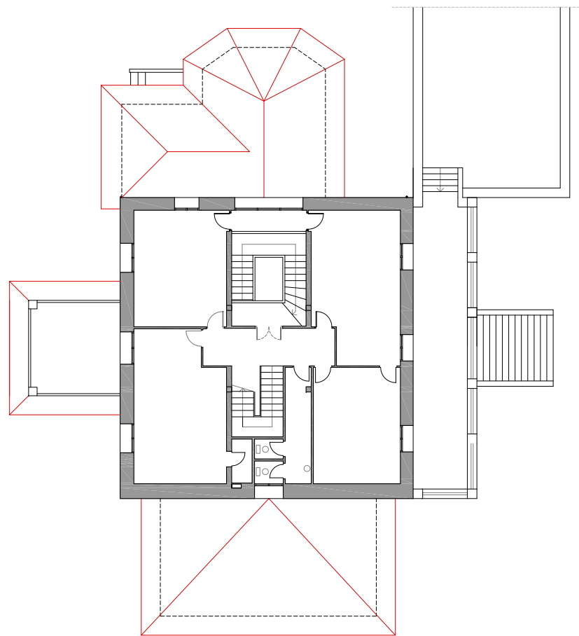
PLANTA PRIMERA
