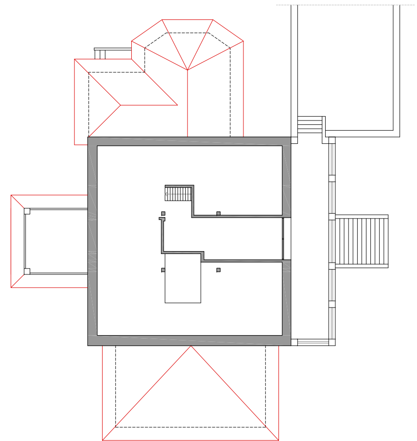
PLANTA BAJOCUBIERTA
