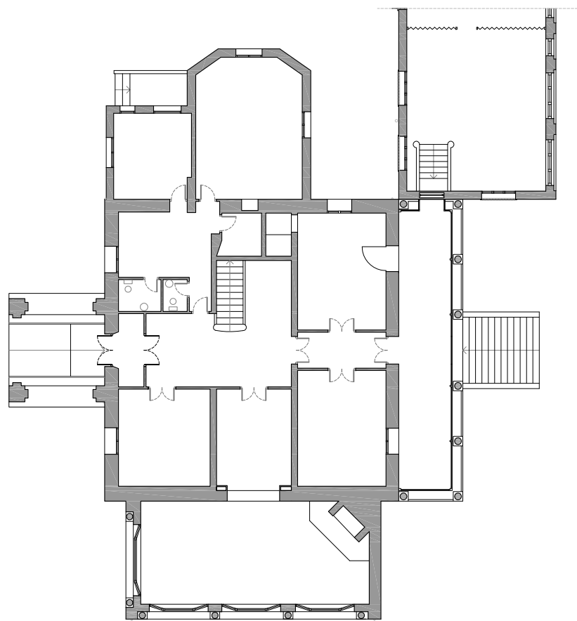
PLANTA BAJA
