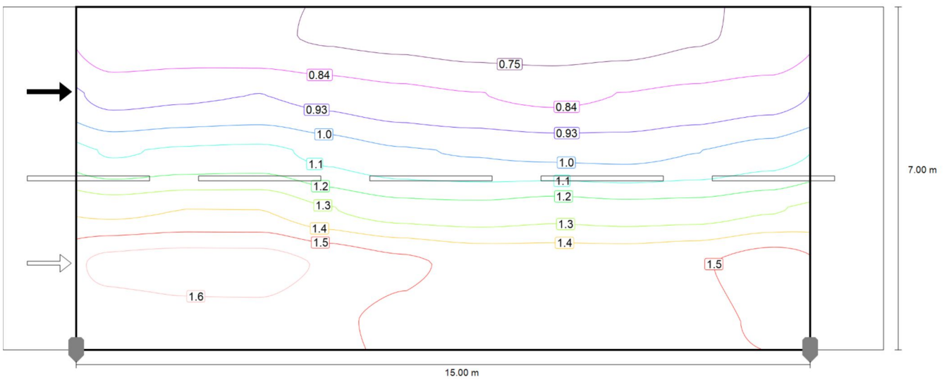
Observador 2: Luminancia para una instalación nueva [cd/m 2 ] (Líneas Isolux)
