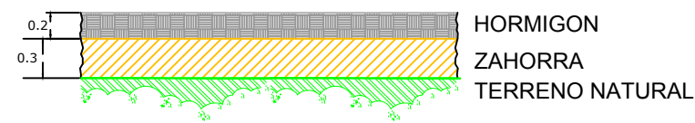
DETALLE SECCION ACCESO A EDAR
