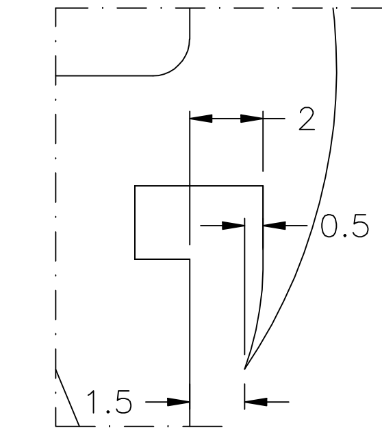
DETALLE Z1 Escala 5:1
