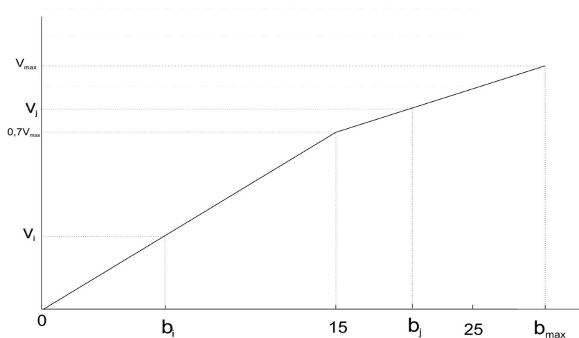
Figura 3: Representación gráfica de as puntuacións se b_{\text{max}} \geq 25 .
