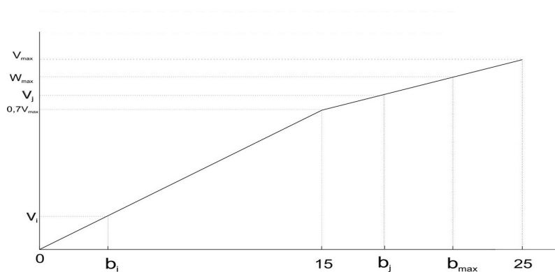
Figura 2: Representación gráfica das puntuacións se 15 \leq b_{max} < 25 .
