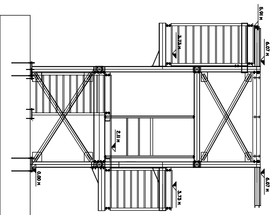
ALZADO 1
