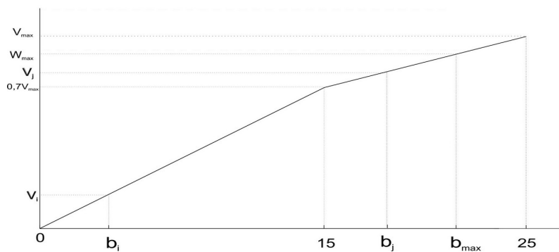
Figura 2: Representación gráfica das puntuacións se 15 \leq b_{max} < 25 .
