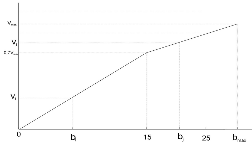
Figura 3: Representación gráfica de as puntuacións se b_{se} \geq 25 .
