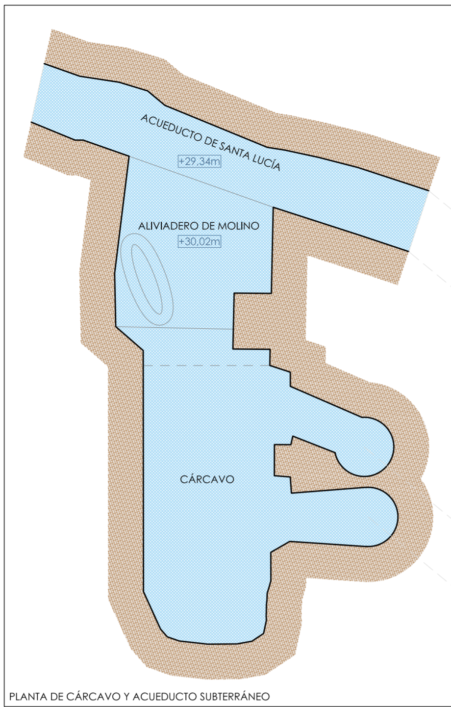
PLANTA DE CÁRCAVO Y ACUEDUCTO SUBTERRÁNEO
