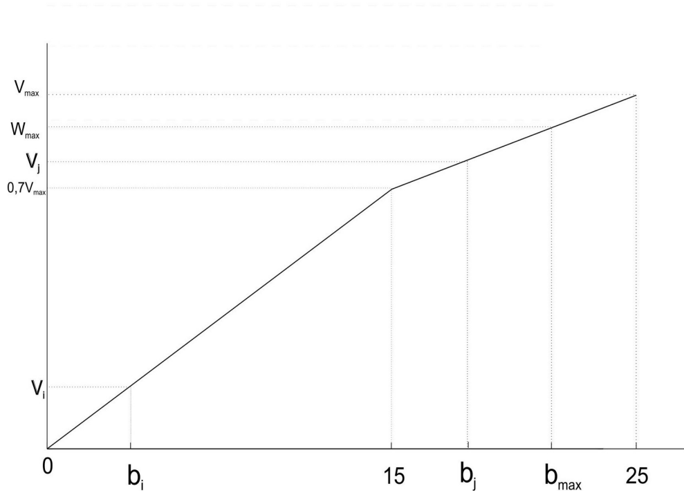
Figura 2: Representación gráfica das puntuacións se b \leq 25 .
