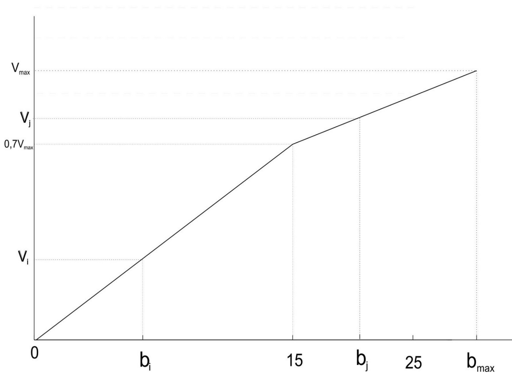
Figura 3: Representación gráfica de as puntuacións se b \geq 25 .
