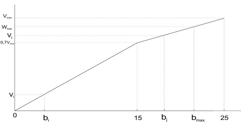
Figura 2: Representación gráfica das puntuacións se 15 \leq b_{max} < 25 .
