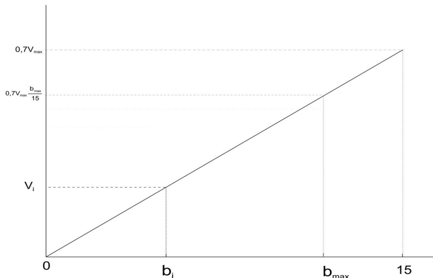
Figura 1: Representación gráfica das puntuacións se b_{max} < 15 .
