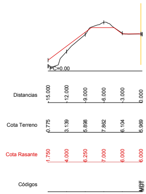
Dp=10.00 P.K.=3440.00 - Perfil N. 57 Z1= 5.969 Z2= 6.000
