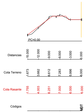
Dp=10.00 P.K.=3380.00 - Perfil N. 51 Z1= 6.000 Z2= 6.000
