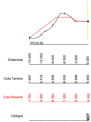
Dp=10.00 P.K.=3500.00 - Perfil N. 63 Z1= 5.940 Z2= 6.000
