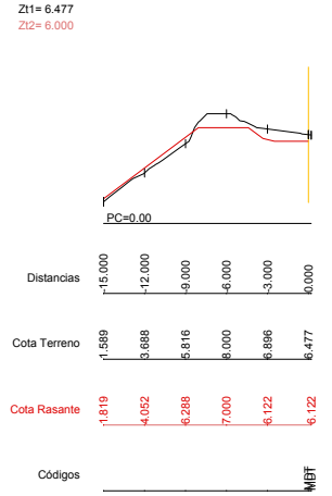
Dp=10.00 P.K.=3120.00 - Perfil N. 25
