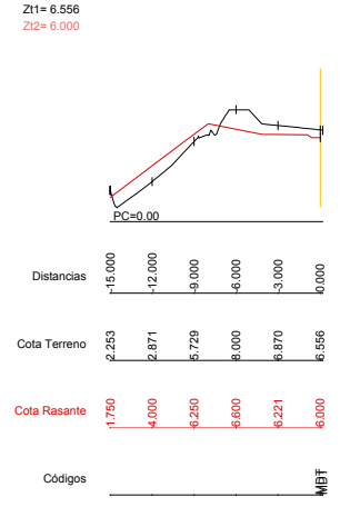
Dp=10.00 P.K.=3150.00 - Perfil N. 28
