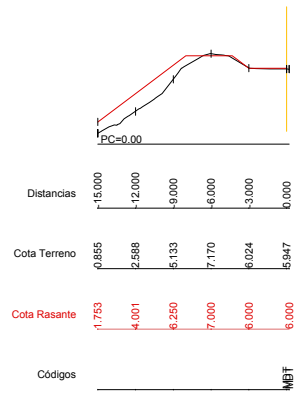
Dp=10.00 P.K.=3420.00 - Perfil N. 55 Z1= 5.947 Z2= 6.000
