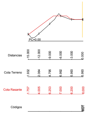
Dp=10.00 P.K.=3400.00 - Perfil N. 53 Z1= 5.993 Z2= 6.000
