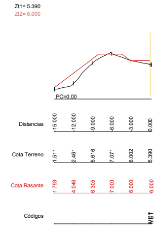
Dp=10.00 P.K.=3260.00 - Perfil N. 39
