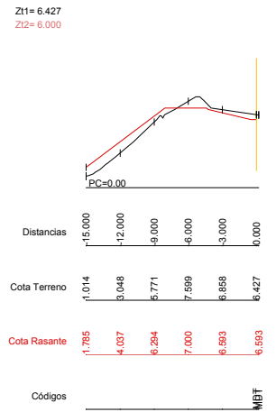
Dp=10.00 P.K.=3140.00 - Perfil N. 27
