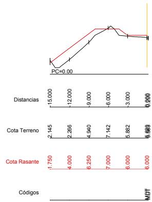
Dp=10.00 P.K.=3330.00 - Perfil N. 46 Z1= 5.620 Z2= 6.000
