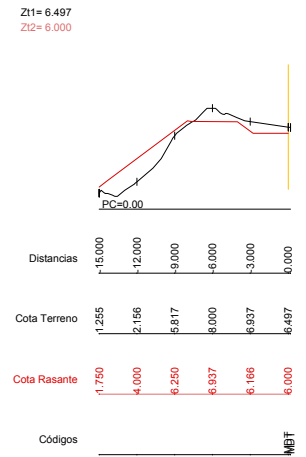
Dp=10.00 P.K.=3170.00 - Perfil N. 30
