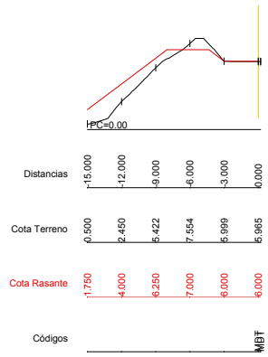
Dp=10.00 P.K.=3460.00 - Perfil N. 59 Z1= 5.965 Z2= 6.000
