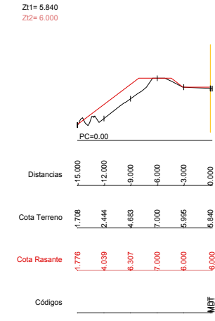
Dp=10.00 P.K.=3280.00 - Perfil N. 41
