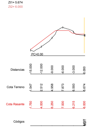
Dp=10.00 P.K.=3240.00 - Perfil N. 37
