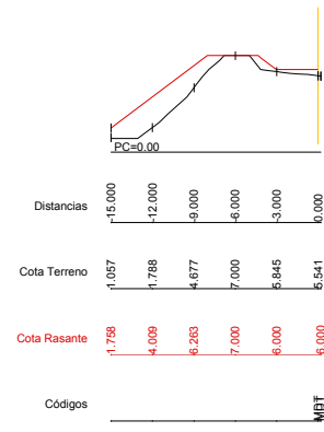
Dp=10.00 P.K.=3320.00 - Perfil N. 45 Z1= 5.541 Z2= 6.000
