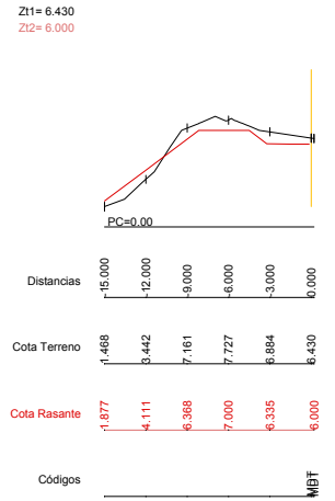
Dp=10.00 P.K.=3130.00 - Perfil N. 26
