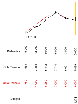
Dp=10.00 P.K.=3350.00 - Perfil N. 48 Z1= 5.489 Z2= 6.000
