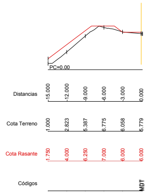
Dp=10.00 P.K.=3340.00 - Perfil N. 47 Z1= 5.779 Z2= 6.000
