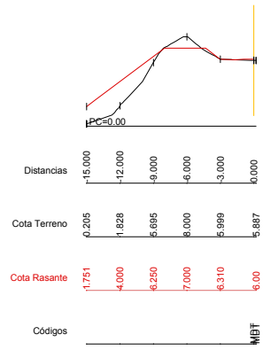
Dp=10.00 P.K.=3430.00 - Perfil N. 56 Z1= 5.893 Z2= 6.000
