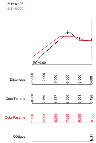
Dp=10.00 P.K.=3200.00 - Perfil N. 33
