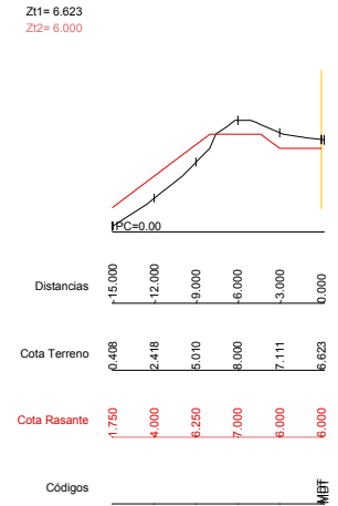
Dp=10.00 P.K.=3190.00 - Perfil N. 32
