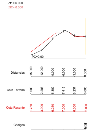
Dp=10.00 P.K.=3250.00 - Perfil N. 38
