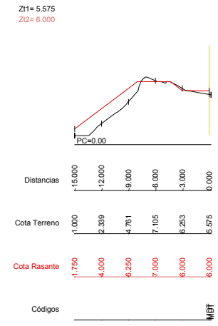
Dp=10.00 P.K.=3230.00 - Perfil N. 36
