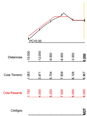
Dp=10.00 P.K.=3360.00 - Perfil N. 49 Z1= 5.967 Z2= 6.000
