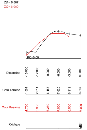
Dp=10.00 P.K.=3090.00 - Perfil N. 22
