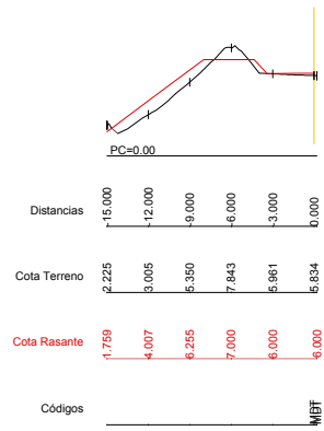
Dp=10.00 P.K.=3390.00 - Perfil N. 52 Z1= 5.834 Z2= 6.000
