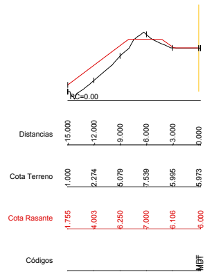
Dp=10.00 P.K.=3410.00 - Perfil N. 54 Z1= 5.973 Z2= 6.000
