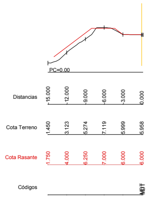
Dp=10.00 P.K.=3470.00 - Perfil N. 60 Z1= 5.958 Z2= 6.000
