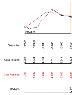
Dp=10.00 P.K.=3300.00 - Perfil N. 43 Z1= 5.528 Z2= 6.000
