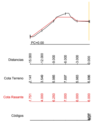
Dp=10.00 P.K.=3370.00 - Perfil N. 50 Z1= 5.886 Z2= 6.000
