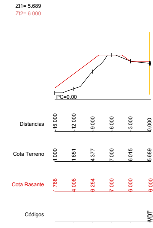
Dp=10.00 P.K.=3290.00 - Perfil N. 42
