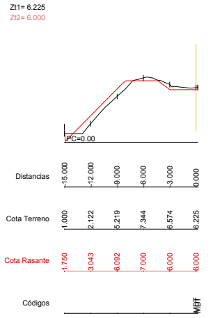
Dp=10.00 P.K.=3100.00 - Perfil N. 23
