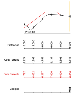
Dp=10.00 P.K.=3310.00 - Perfil N. 44 Z1= 5.545 Z2= 6.000
