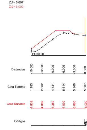
Dp=10.00 P.K.=3270.00 - Perfil N. 40
