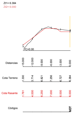
Dp=10.00 P.K.=3110.00 - Perfil N. 24
