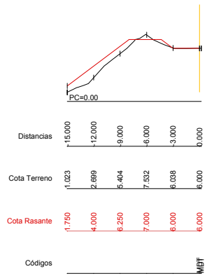
Dp=10.00 P.K.=3480.00 - Perfil N. 61 Z1= 6.000 Z2= 6.000
