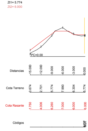
Dp=10.00 P.K.=3210.00 - Perfil N. 34
