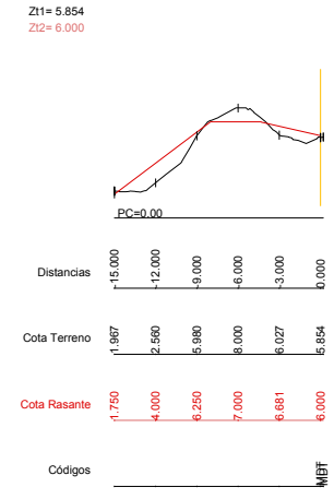
Dp=10.00 P.K.=3220.00 - Perfil N. 35
