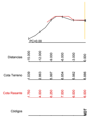
Dp=10.00 P.K.=3450.00 - Perfil N. 58 Z1= 5.886 Z2= 6.000
