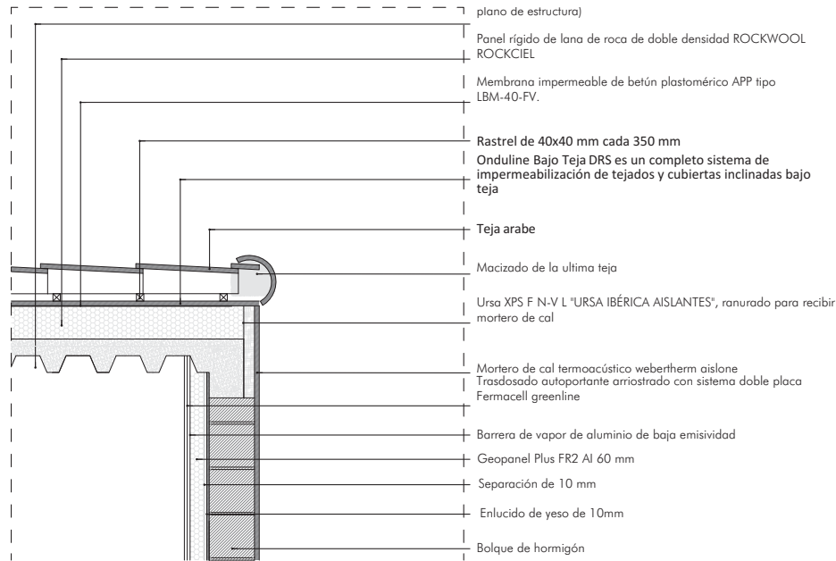
DET 8
