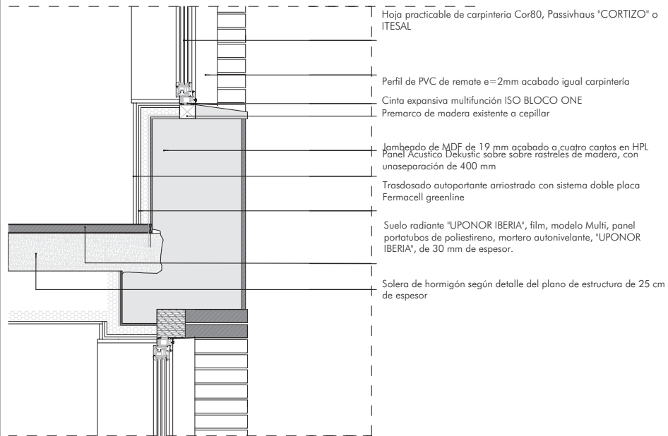
DET 3 Encuentro Losa con fachada DET 3 1:10 Encuentro Losa con fachada 1:10
