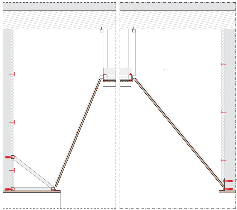
DET 6 Falso Techo Pasillo 1:10
