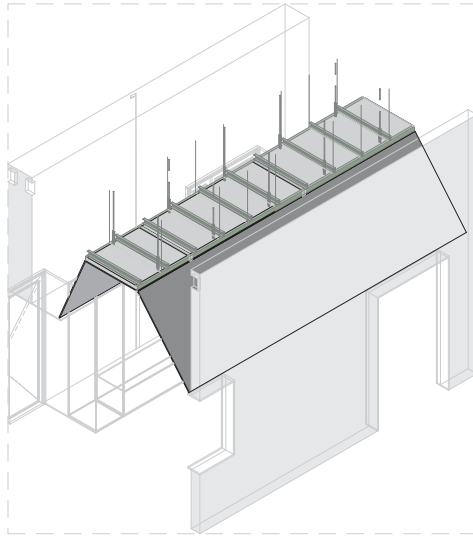
Falso techo Estructura 1:50
