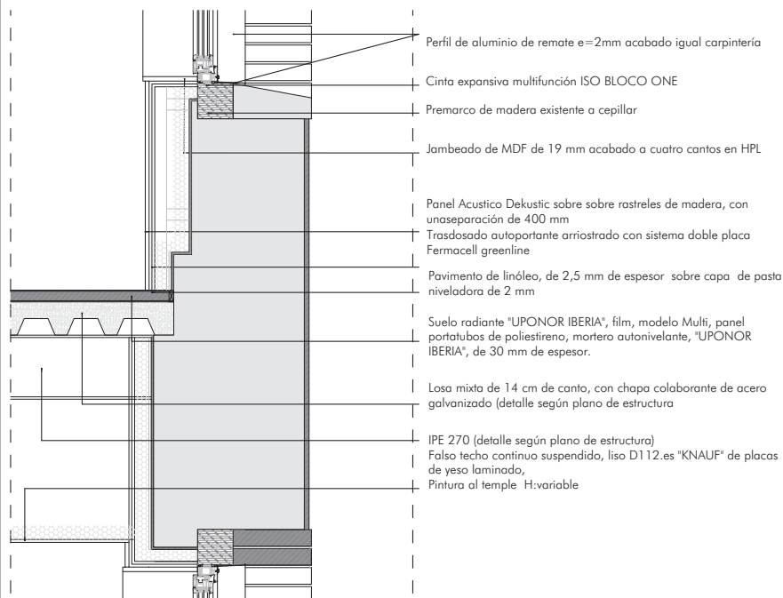
DET 4 Ventana DET 4 1:10
