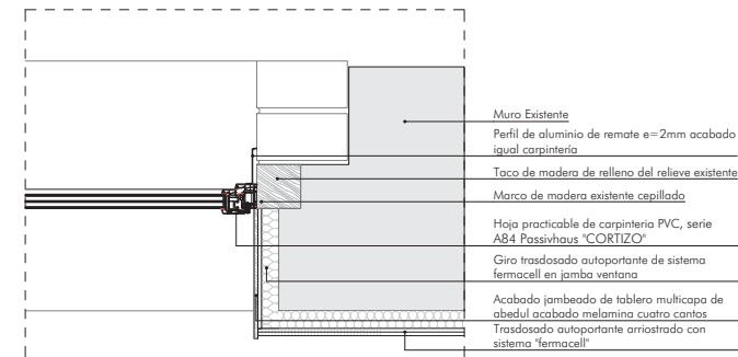
CARPINTERIA TIPO SECCIÓN HORIZONTAL
