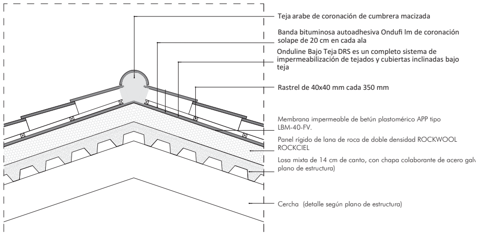
DET 1 Cubierta - Cumbre 1:10
