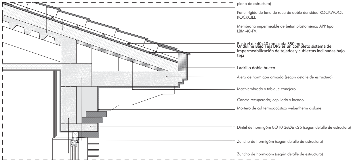
DET 2 Cubierta - Alero 1:10
