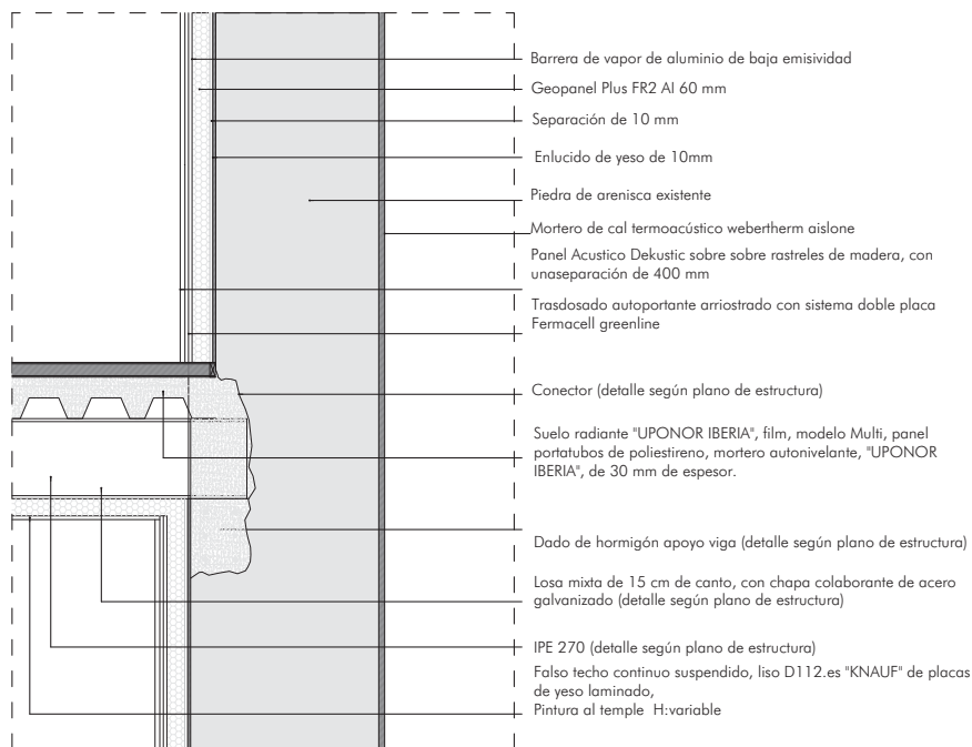
DET 4 Parte placa DET 4 1:10
