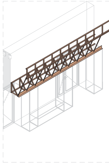
Bastidores Mueble 1:50
