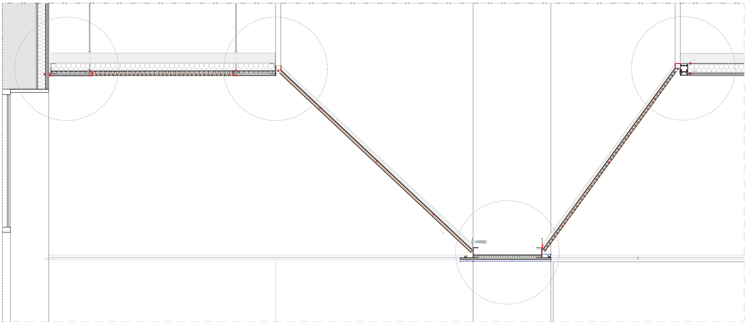
DET 7 Falso Techo. Pasillo Aseos y Ascensor 1:10
