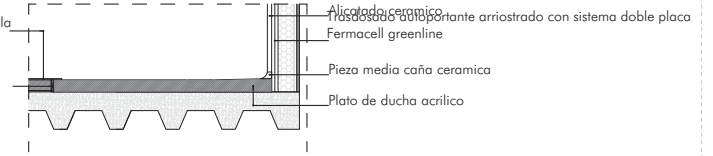
Detalle Ducha 1:10
