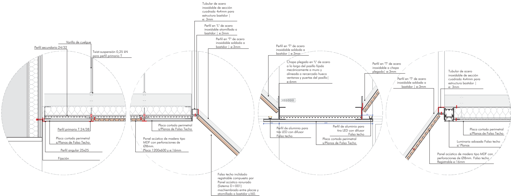
DET 7 Falso Techo. Pasillo Aseos y Ascensor 1:10
