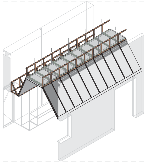
Falso techo 1:50
