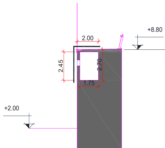
Sección tipo Tramo 1 y perfil tipo 1
