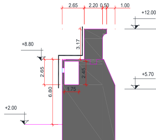
Sección tipo Tramo 2 y 3 y perfil tipo 2
