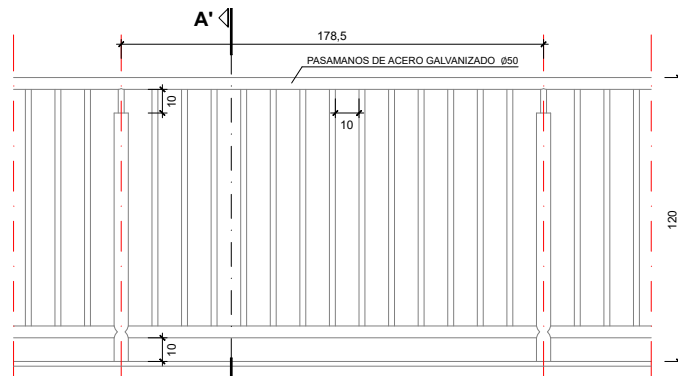
ALZADO
