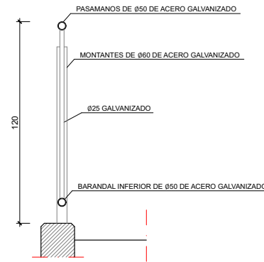
SECCIÓN A-A
