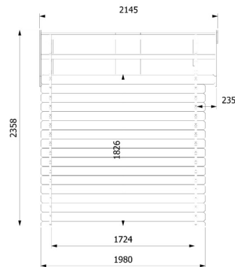
ALZADO LATERAL
