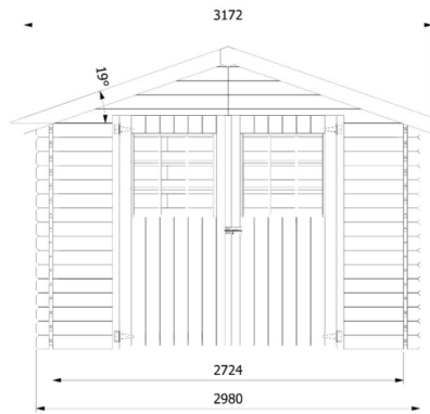
ALZADO FRONTAL
