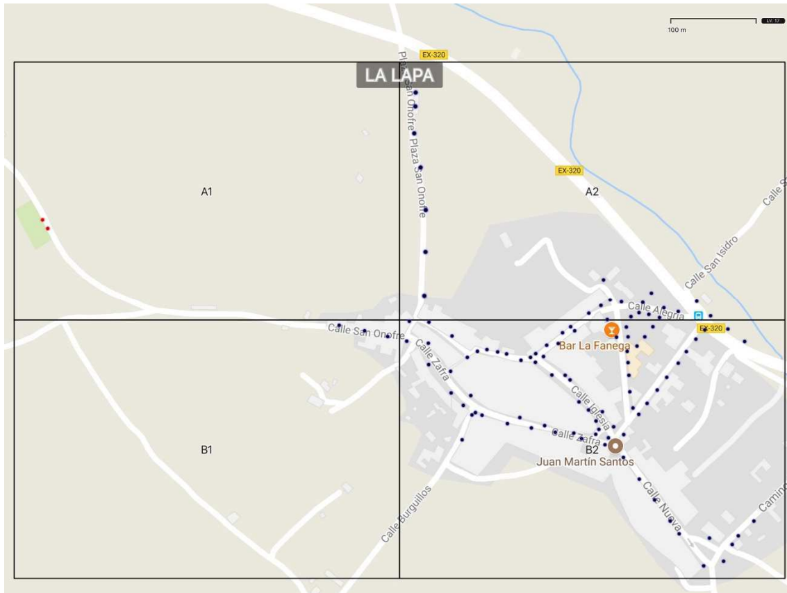
IMAGEN 1. DISTRIBUCIÓN DE TODAS LAS LUMINARIAS EXISTENTES: EN AZUL SON LUMINARIAS RESULTANTES EN LED, EN ROJO SIN ACTUACIÓN PREVISTA (LA LAPA)
