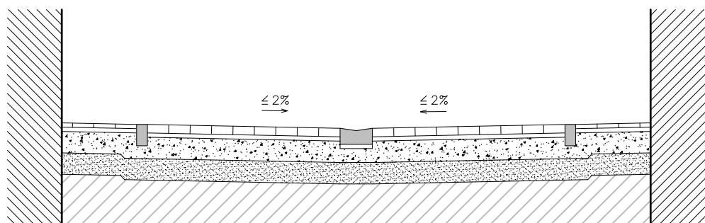
SECCION A
