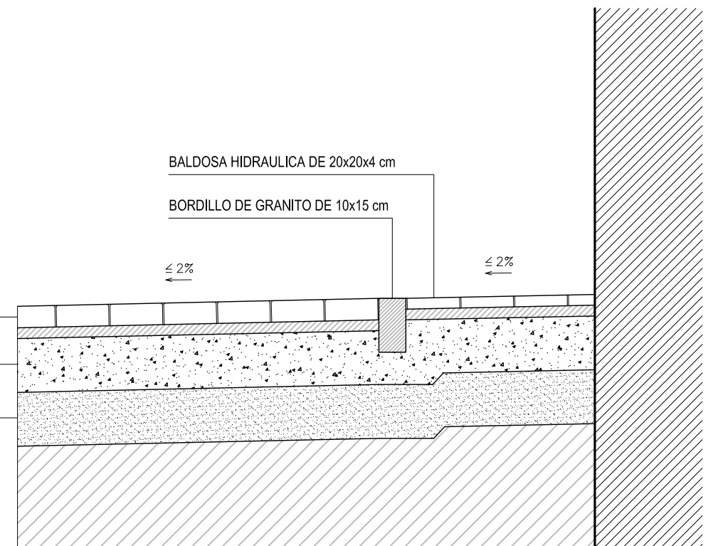
DETALLE B
