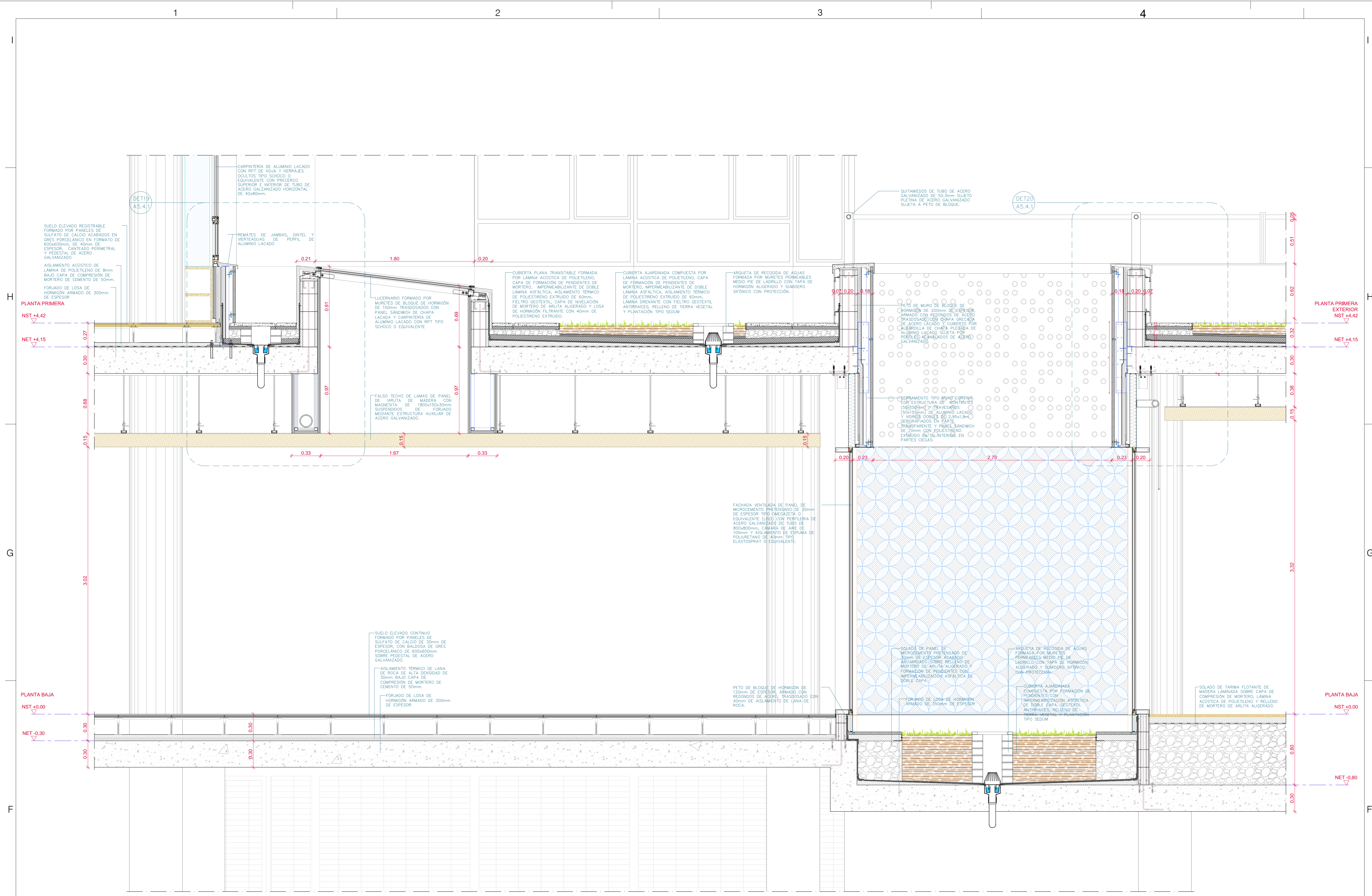
SECCIÓN LUCERNARIO - SALÓN DE ACTOS
