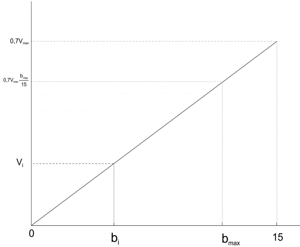
Figura 1: Representación gráfica das puntuacións se b_{max} < 15 .
