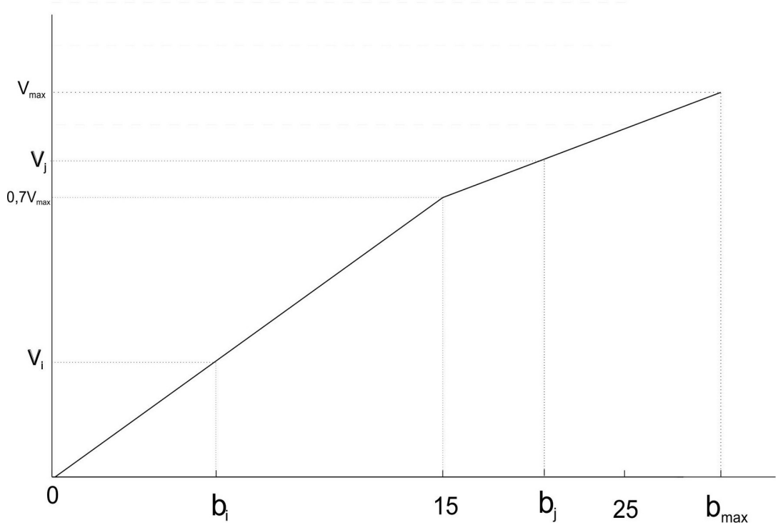
Figura 3: Representación gráfica das puntuacións se b_{max} \geq 25 .
