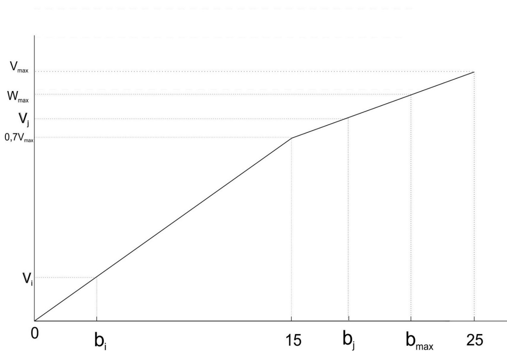
Figura 2: Representación gráfica das puntuacións se 15 \leq b_{max} < 25 .
