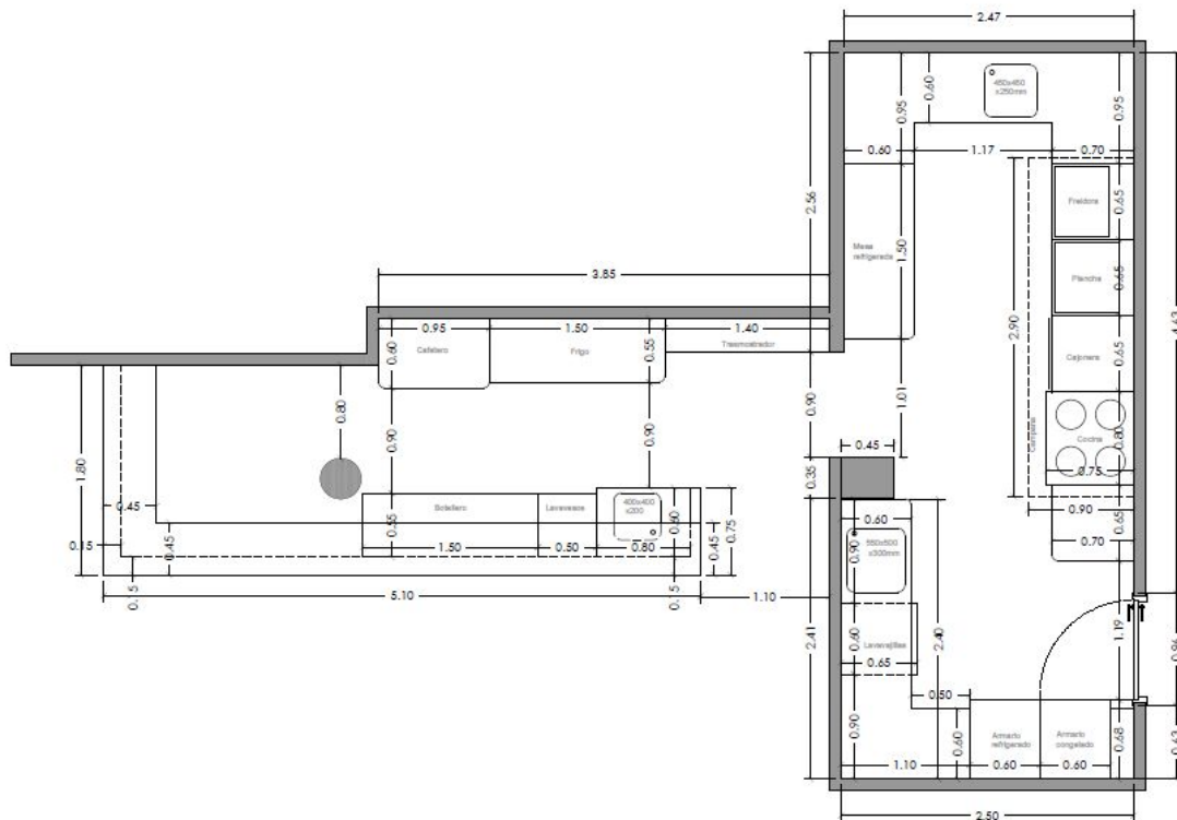
Zona Barra y Cocina del Salón Social. Distribución de equipamiento (sin escala)
