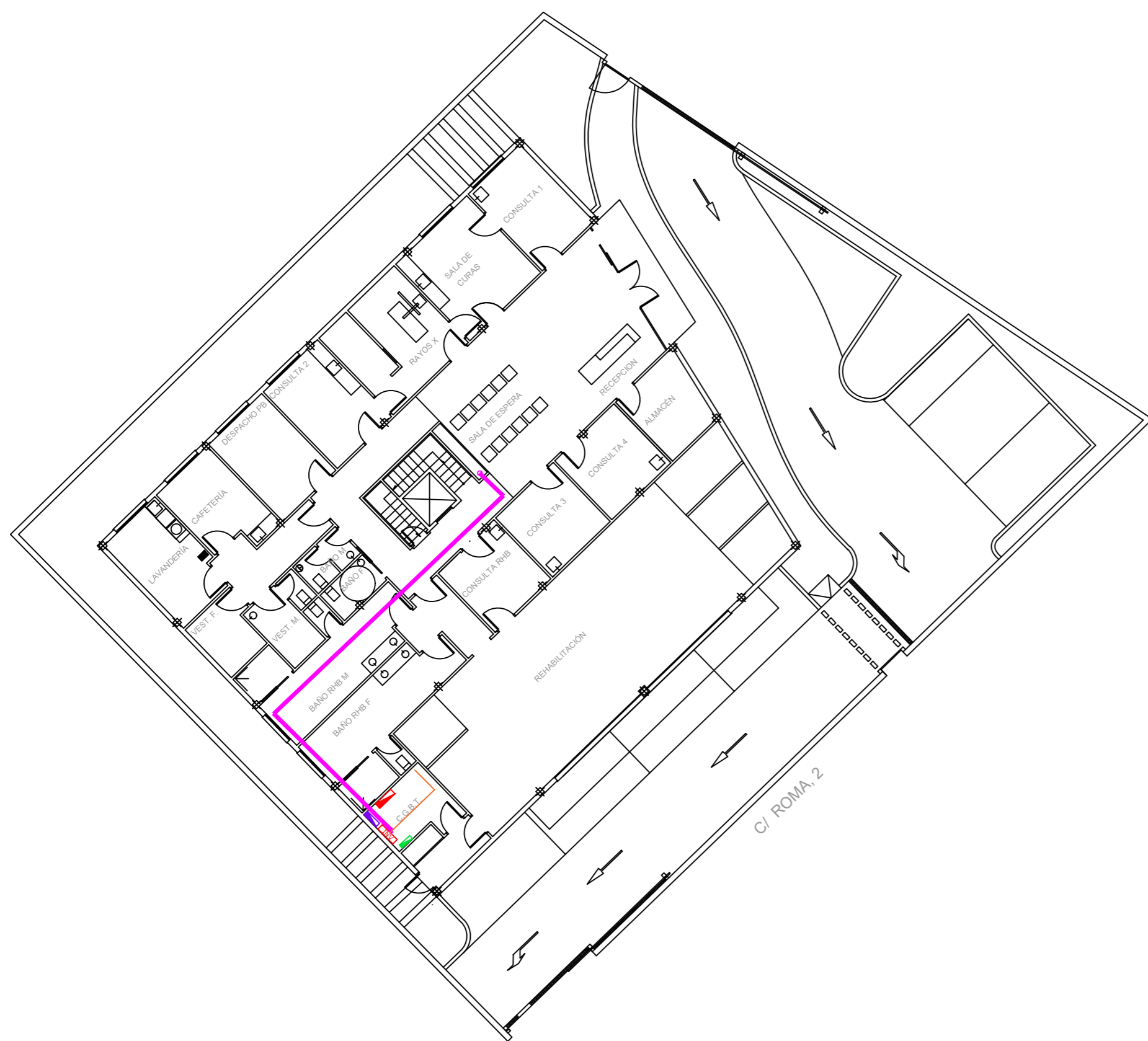
PLANTA BAJA
